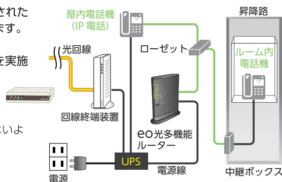
無停電電源装置 (UPS) 設置例
